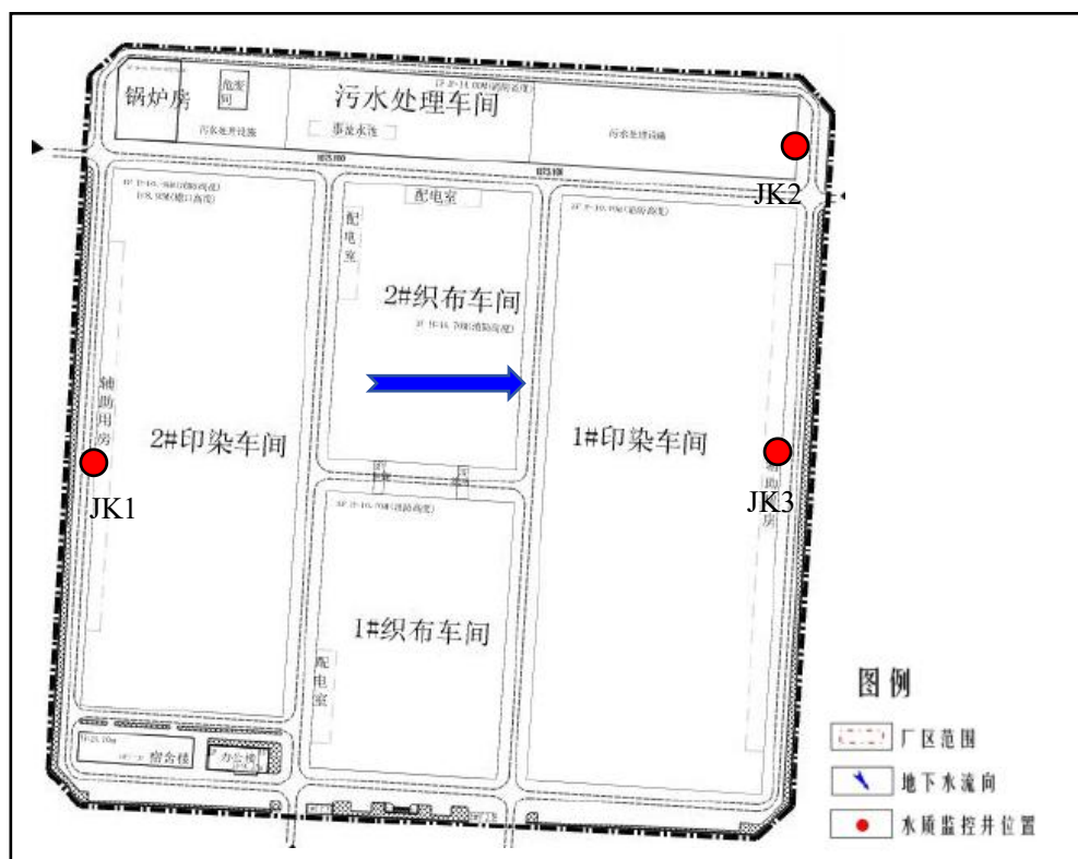
图 5.3-15 本项目监控井布设图
