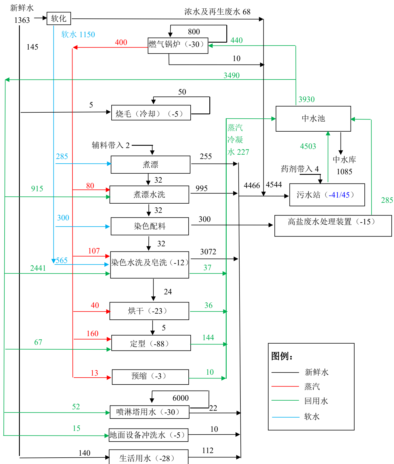
图 3.7-1 本项目给排水平衡图 单位：m³/d
