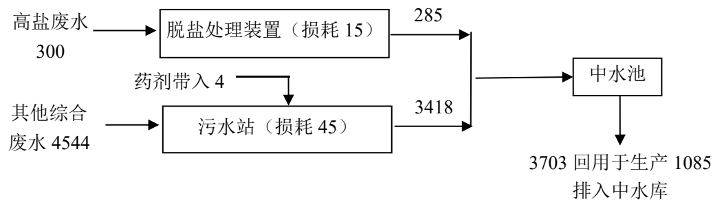
图 3.8-1 本项目废水处理示意图 单位：m 3 /d
