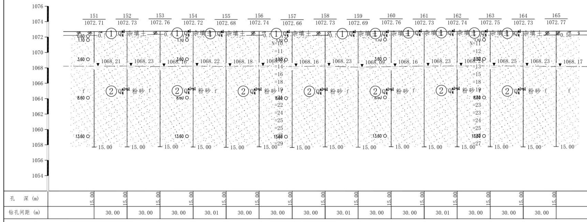
图 5.4-1 工程地质剖面图
