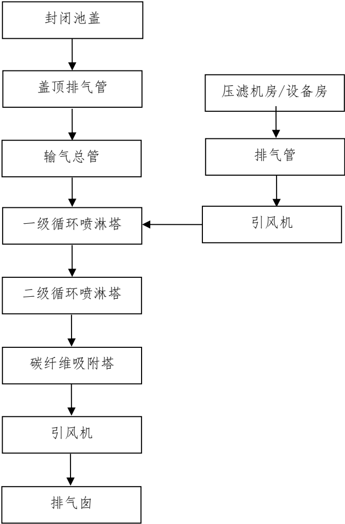
图 6.2-5 废气处理工艺流程图
