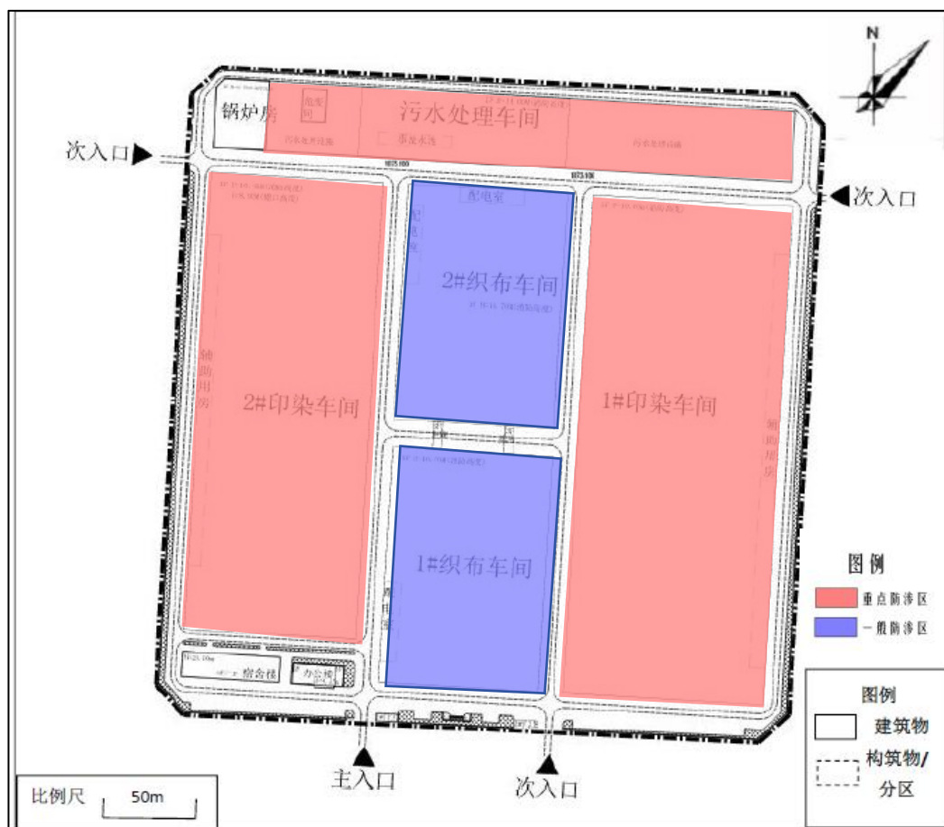
图 5.3-10 厂区防渗分区图
