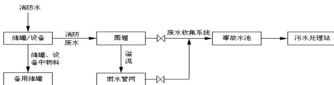
图 5.3-2 燃烧时消防废水传输图
