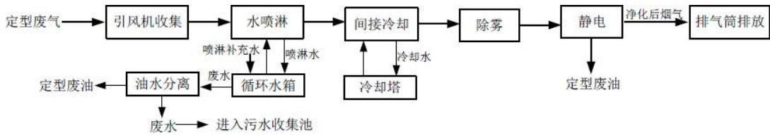
图 6.2-1 定型废气处理工艺流程图
