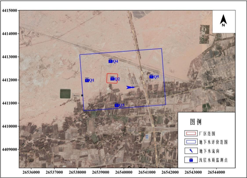
图 4.3-1 地下水现状监测点位图
